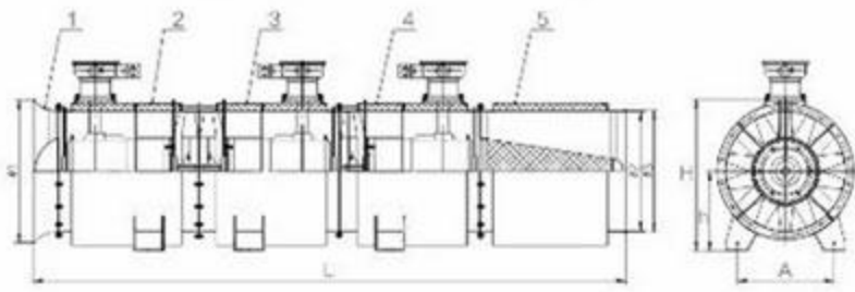
1. 集流器 2. 一级主机 3. 二级主机 4. 三级主机 5. 叶轮器
